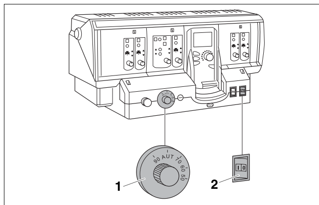
Fig. 3 Conectar la instalacin de calefaccin (Logamatic 4000)
